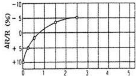
&lt;압축응력에 따른 반발경도 보정곡선&gt;
